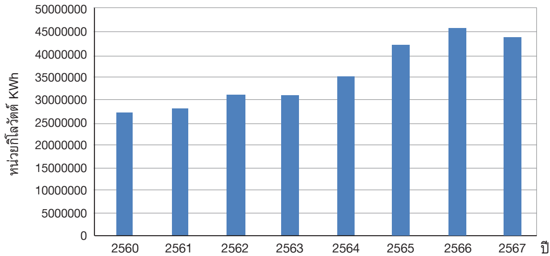
ปริมาณไฟฟ้าที่ผลิตได้จากโครงการกักเก็บก๊าซมีเทน ตั้งแต่ปี 2560 - 2567
