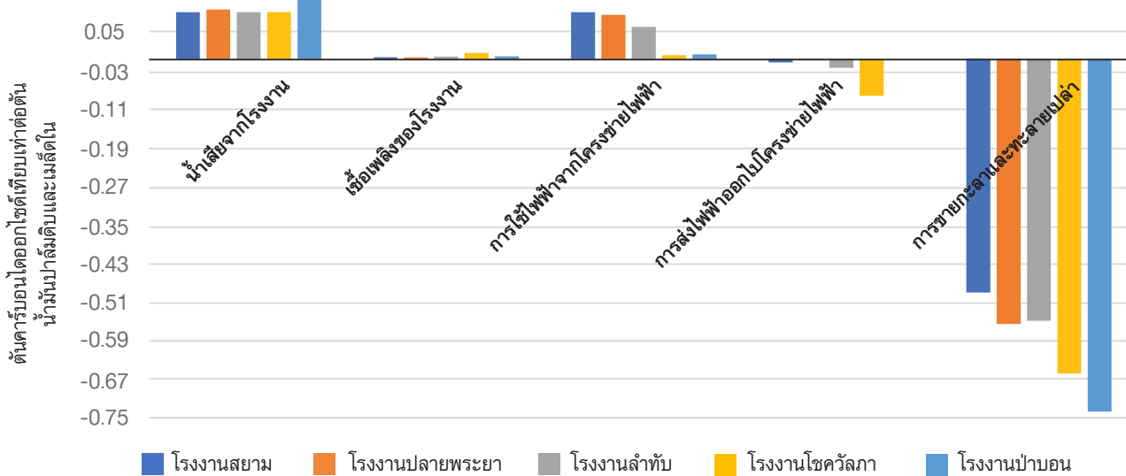
การปล่อยก๊าซเรือนกระจกของโรงงานยูนิวานิช ปี 2567 (MTCO 2 e/MT CPO&PK Ex-Factory)
